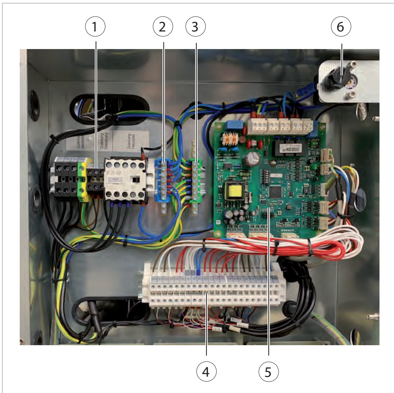
Abb. 1: Schaltkasten
