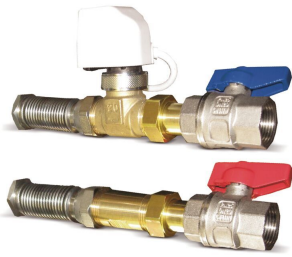
RK 2-Wege-Ventilbaugruppe, kpl., KWD 20-50/25-55 (EC)
