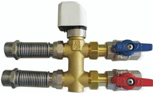
RK 3-Wege-Ventilbaugruppe, kpl. KWD 20-50/25-55 (EC) - VB10.1
