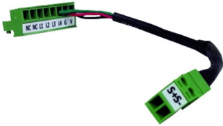
SolarEdge S0 Zähler Adapterkabel
