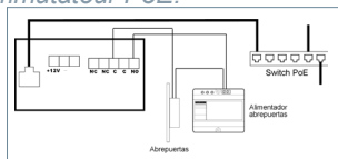
Schéma de base utilisant un commutateur PoE.
