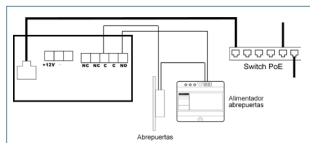
Grundschemata mit PoE-Switch.
