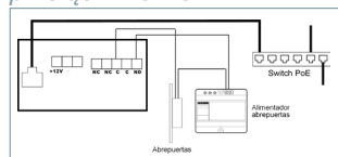
Podstawowy schemat przy użyciu przełącznika PoE.
