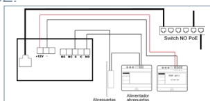
Schéma de base utilisant un commutateur non PoE.
