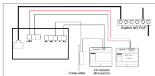
Grundschemata mit Nicht-PoE-Switch.
