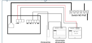
Schemat podstawowy przy użyciu przełącznika innego niż PoE.
