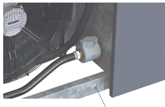
Anschlussmöglichkeit Blitzschutz
