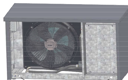
Vier Transportöffnungen (jeweils zwei auf Ansaug- und Ausblasseite)
