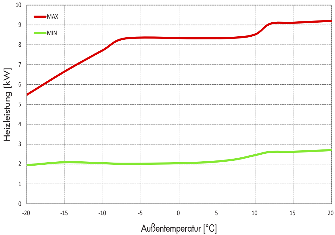
Heizleistung bei Vorlauftemperaturen von 35 °C
