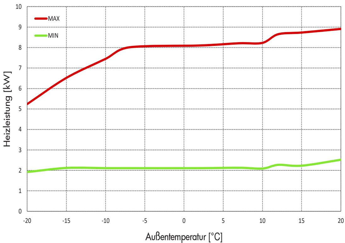
Heizleistung bei Vorlauftemperaturen von 45 °C
