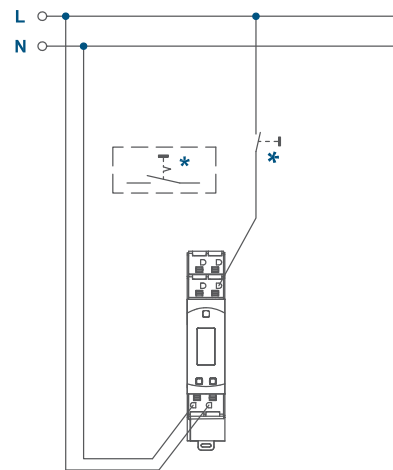
Anschluss von Tastern/Schaltern (Eingänge):
