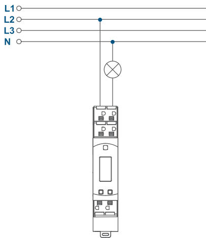
Anschluss von verschiedenen Lasten (Ausgänge):
