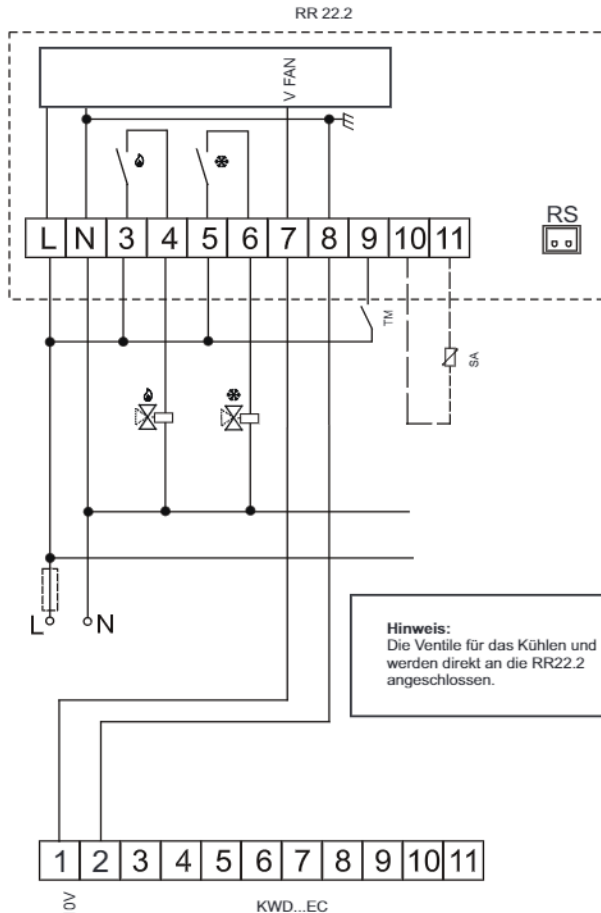
RR 22.2 mit KWD...EC, Zweileiter-System (Beispiel)
