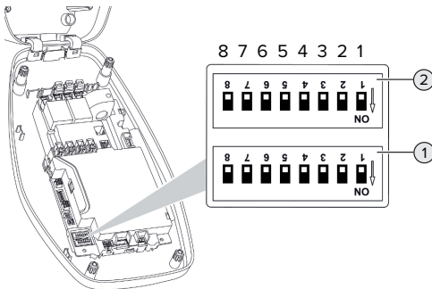
Fig. 11: Interruptores DIP (estado de entrega)
