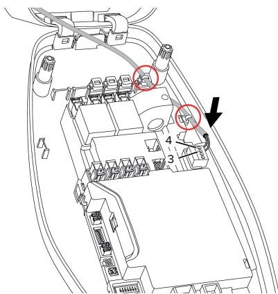
Fig. 12: Tilslutning downgrade-indgang
