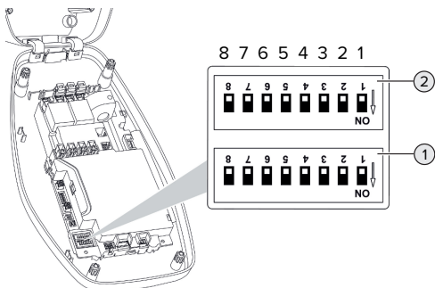
Fig. 11: DIP-brytere (utlevert tilstand)
