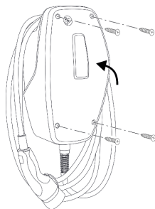
Obr. 16: Zavření výrobku
