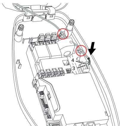
Fig. 12: Anslutning av downgrade-ingång
