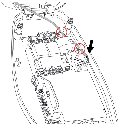
Fig. 12: Ligação da entrada "downgrade"
