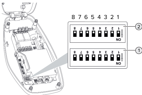
11. Ábra: DIP kapcsoló (gyári állapot)
