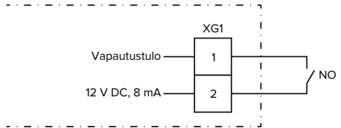
Kuva 15: PeriaatekytKentäkaavio: vapautustulo
