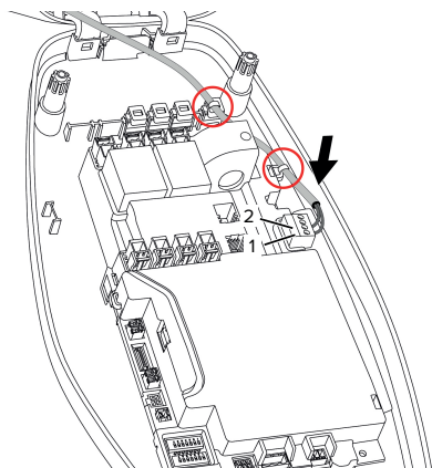
Pav. 14: Leidimo įėjimo jungtis
