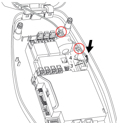
Afb. 12: Aansluiting downgrade-ingang
