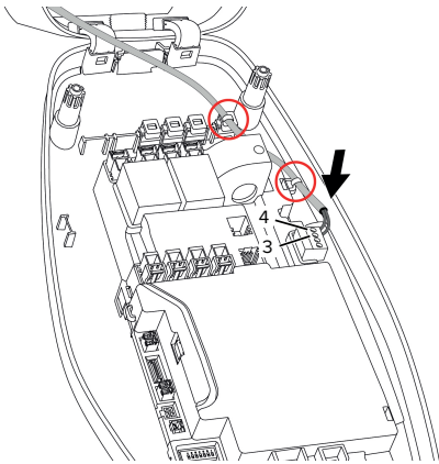
Pav. 12: Žeminimo jėjimo jungtis
