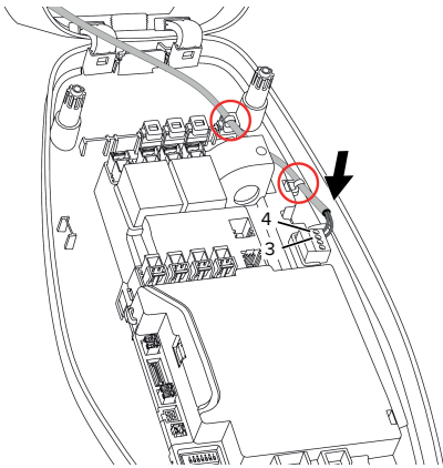
Obr. 12: Připojení vstupu Downgrade
