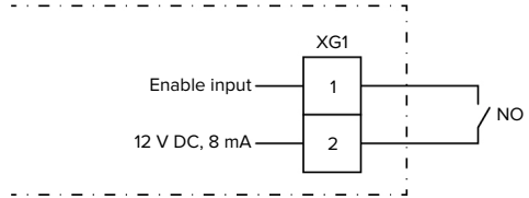
Fig. 15: Schematic circuit diagram: Enable input
