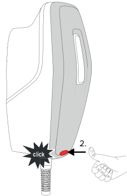
Fig. 19 : Monter le cache frontal - 2
