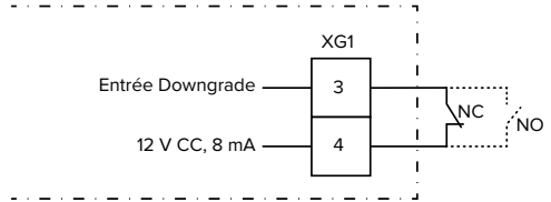
Fig. 13 : Schéma de principe : raccordement d'un contact électrique externe (réglage par défaut : NO)
