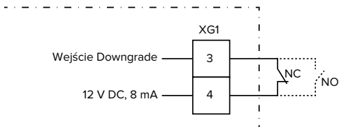
Ilustr. 13: Schemat blokowy: podłączenie zewnętrznego styku przełączającego (ustawienie standardowe: NO)
