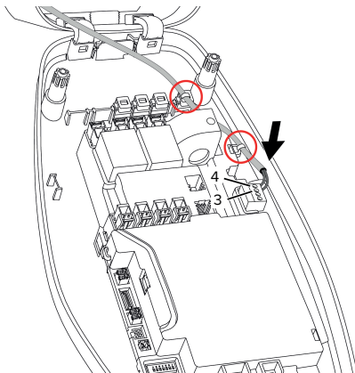
Fig. 12 : Raccordement de l'entrée Downgrade
