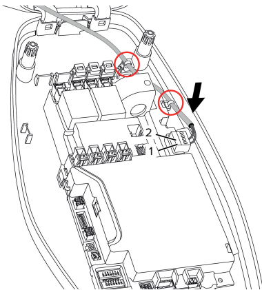
Fig. 14: Anslutning av aktiveringsingång
