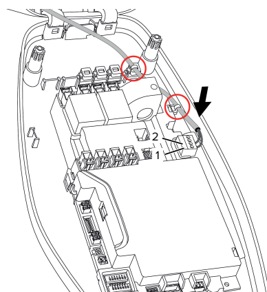
Fig. 14: Collegamento ingresso di abilitazione
