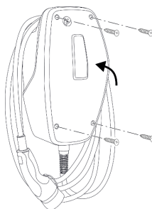
Fig. 16: Fechar o produto
