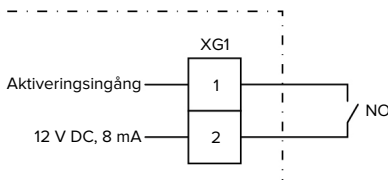
Fig. 15: Principkopplingschema: Aktiveringsingång
