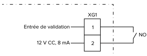
Fig. 15 : Schéma de principe : Entrée de validation
