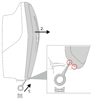
Fig. 4: Lossa frontkåpan
