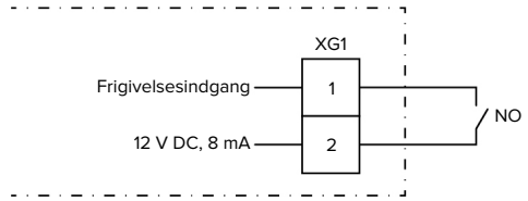
Fig. 15: Principskema: Frigivelsesindgang
