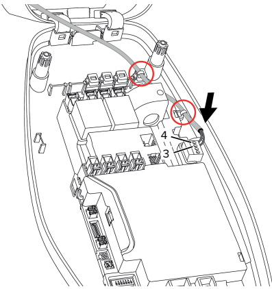
Kuva 12: Downgrade-tulon liitäntä
