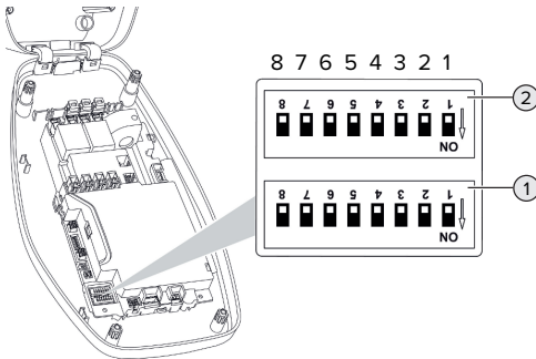
Afb. 11: Dipschakelaar (uitleveringstoestand)
