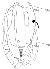
Fig. 16 : Fermeture du produit
