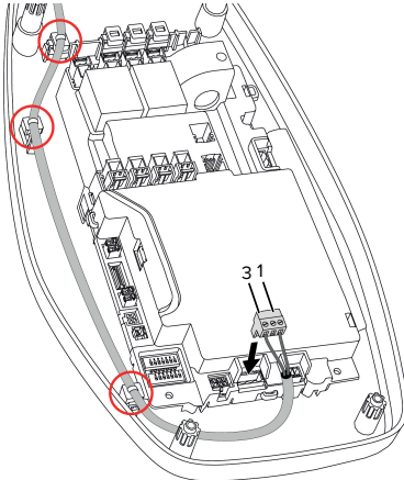
9. Ábra: Söntkioldó csatlakoztatása
