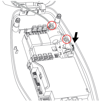
Εικ. 12: Σύνδεση εισόδου περιορισμού ισχύος
