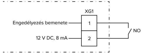
15. Ábra: Elvi kapcsolási rajz: Engedélyezés bemenete
