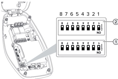
Fig. 11: Conmutadores DIP (estado de entrega)
