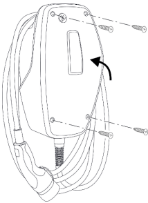
Fig. 16: Stenge produktet
