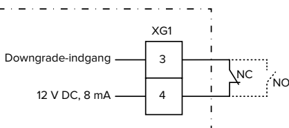
Fig. 13: Principskema: Tilslutning af en ekstern omskifterkontakt (standardindstilling: NC)
