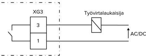
Kuva 10: Periaatekytkentäkaavio: ulkoisen työvirrän laukaisijan liitännät
