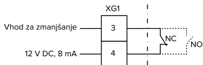
sl. 13: Osnovna vezalna shema: Priključitev zunanega preklopnega kontakta (standardna nastavev: NO)
