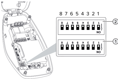
Obr. 11: DIP přepínače (stav při dodání)
