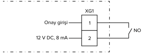
Şek. 15: Prensipsel devre şeması: Onay girişi
