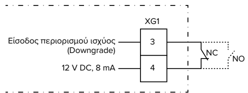
Εικ. 13: Διάγραμμα συνδεσμολογίας: Σύνδεση εξωτερικής επαφής μεταγωγής (βασική ρύθμιση: NO)
