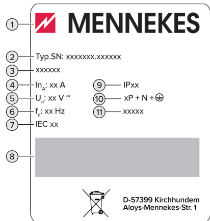
Ilustr. 1: Tabliczka znamionowa produktu (wzór)
