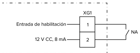
Fig. 15: Esquema de principio: Entrada de habilitación
