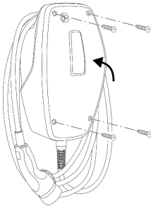
Fig. 16: Lukke produktet
