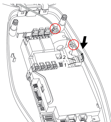
Fig. 14 : Raccordement de l'entrée de validation
