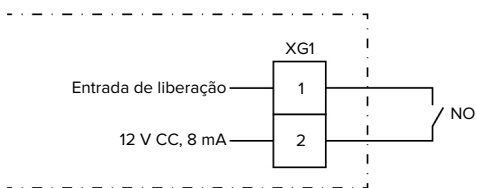
Fig. 15: Esquema de princípio: Entrada de liberação
