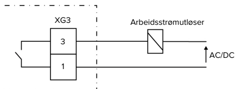
Fig. 10: Prinsipielt koblingskjema: Tilkobling av en ekstern arbeidsstrømutløser
