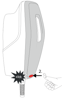
Fig. 19: Montaggio della cover anteriore - 2
