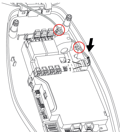
14. Ábra: Engedélyezési bemenet csatlakozás
