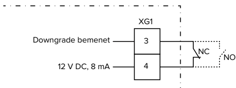
13. Ábra: Elvi kapcsolási rajz: Külső kapcsolóérintkező csatlakoztatása (normál beállítás: NO)
