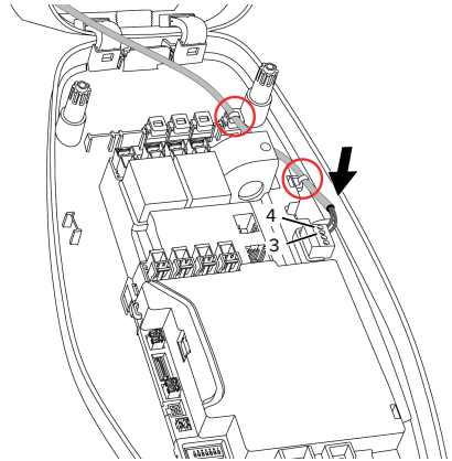
Fig. 12: Conexión entrada Downgrade
