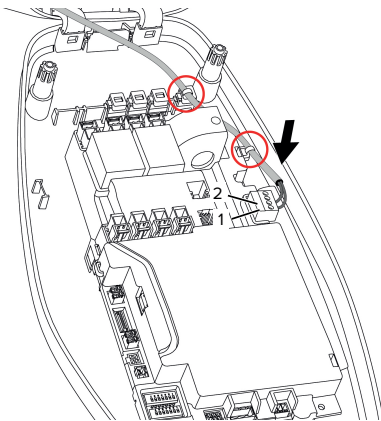
Abb. 14: Anschluss Freigabe-Eingang
