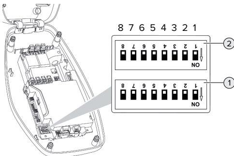
Εικ. 11: Διακόπτες DIP (κατάσταση κατά την πα-ράδοση)
