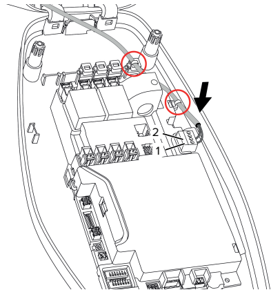
Ilustr. 14: Zaciski przyłączeniowe – wejście zwalniające
