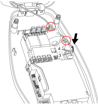
Abb. 12: Anschluss Downgrade-Eingang
