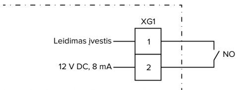
Pav. 15: Principinė sujungimo schema: leidimo įėjimas
