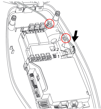
Afb. 14: Aansluiting vrijgaveingang
