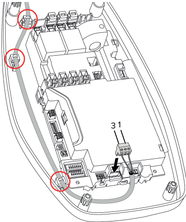
Fig. 9: Tilkobling av arbeidsstrømutløser
