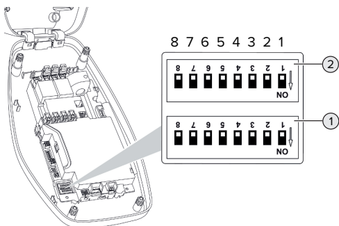
Ilustr. 11: Przełącznik DIP (stan w momencie dostawy)
