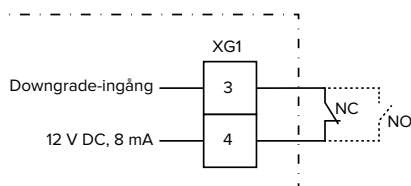
Fig. 13: Principkopplingschema: Anslutning av en extern brytarkontakt (standardinställning: NO)
