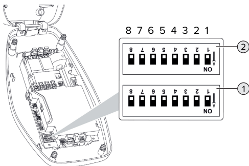
Fig. 11: DIP-kontakter (udleveringstilstand)
