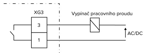
Obr. 10: Základní schéma zapojení: připojení externího vypínače pracovního proudu
