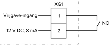
Afb. 15: Principe-schakelschema: Vrijgaveingang
