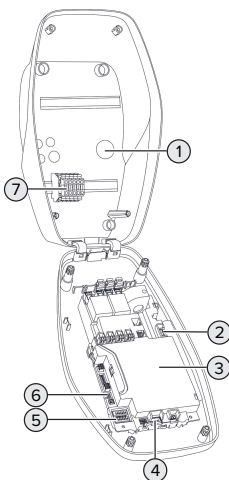
Εικ. 3: Εσωτερική όψη
