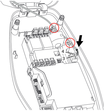
Şek. 12: Downgrade girişi bağlantısı
