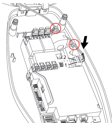
Fig. 14: Ligação da entrada de liberação
