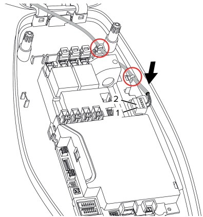
Fig. 14: Conexión entrada de habilitación
