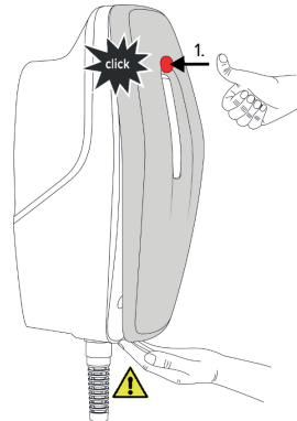
Εικ. 18: Τοποθέτηση του μπροστινού καλύμματος - 1
