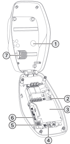
Fig. 3: Indvendig
