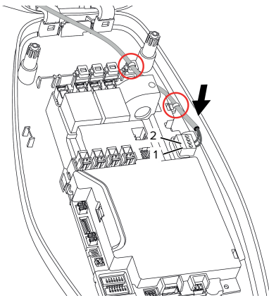
Fig. 14: Tilkobling tilgangsinngang
