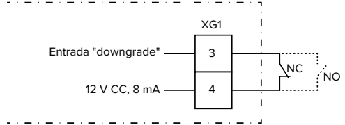
Fig. 13: Esquema de princípio: ligação de um contacto de comutação externo (configuração padrão: NO)
