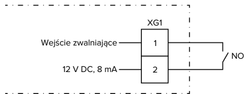
Ilustr. 15: Schemat blokowy: Wejście zwalniające
