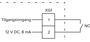
Fig. 15: Prinsipielt koblingsskjema: Tilgangsinngang
