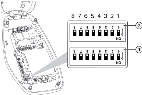
Kuva 11: DIP-kytkin (toimitustila)
