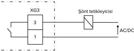
Şek. 10: Prensipsel devre şeması: Harici bir şönt tetikleyicisinin bağlanması
