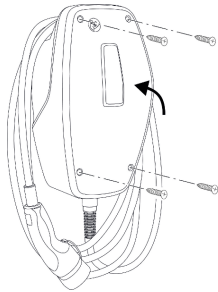
Kuva 16: Tuotteen sulkeminen
