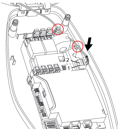
Fig. 14: Tilslutning frigivelsesindgang
