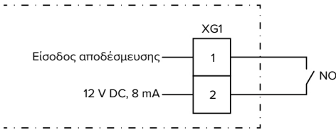
Εικ. 15: Διάγραμμα συνδεσμολογίας: Είσοδος αποδέσμευσης
