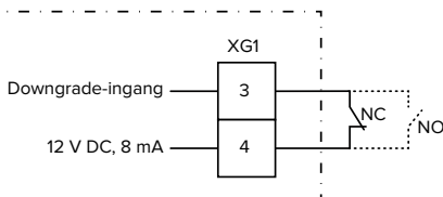
Afb. 13: Principe-schakelschema: Aansluiting van een extern schakelcontact (standaardinstelling: NO)
