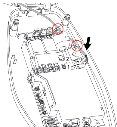
Obr. 14: Připojení uvolňovacího vstupu
