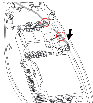
Şek. 14: Onay girişi bağlantısı
