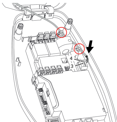
12. Ábra: Downgrade bemenet csatlakoztatása
