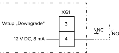
Obr. 13: Základní schéma zapojení: Připojení externího spínacího kontaktu (standardní nastavení: NO)
