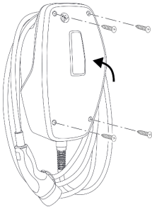
Fig. 16: Stänga produkten
