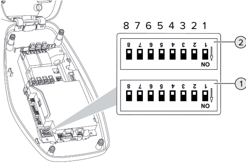
Şek. 11: DIP şalteri (teslimattaki durum)
