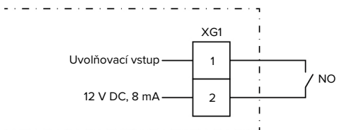
Obr. 15: Základní schéma zapojení: uvolňovací vstup
