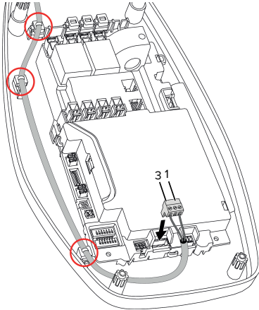
Kuva 9: Työvirtalaukaisijan liitännät
