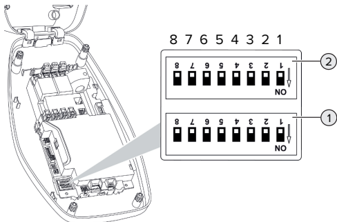
sl. 11: DIP-stikalo (stanje ob dobavi)
