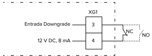
Fig. 13: Esquema de principio: Conexión de un contacto de conmutación externo (ajuste estándar: NO)
