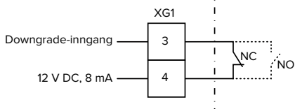
Fig. 13: Prinsipielt koblingsskjema: tilkobling av en ekstern bryterkontakt (standardinnstilling: NO)
