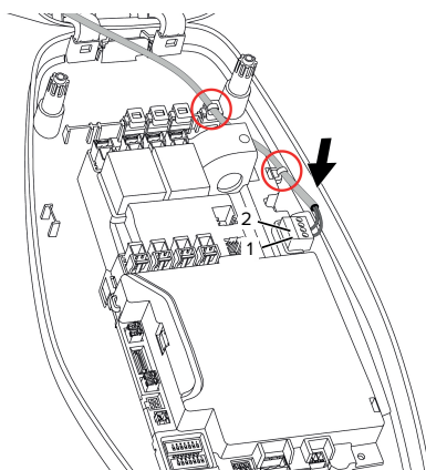
Εικ. 14: Δύνδεση εισόδου αποδέσμευσης
