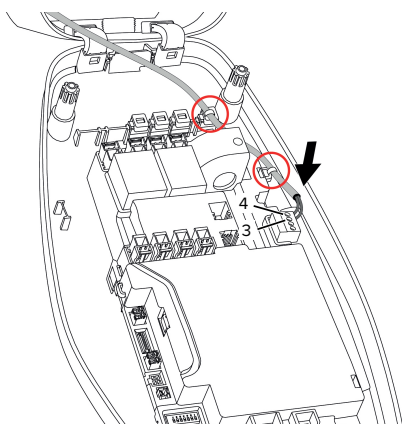
sl. 12: Priključek vhoda za zmanjšanje
