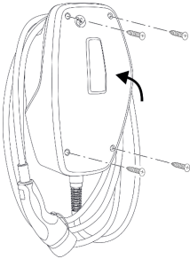
sl. 16: Zapiranje izdelka
