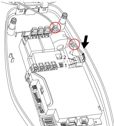
Kuva 14: Liitäntä vapautustulo
