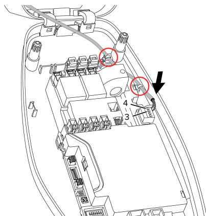
Ilustr. 12: Przyłącze wejścia Downgrade
