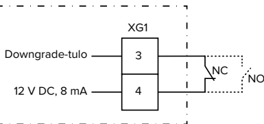
Kuva 13: Periaatekytkentäkaavio: ulkoisen kytkentäkontaktin liitäntä (vakioasetus: NO)
