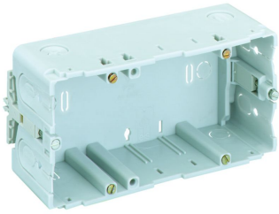
SPELSBERG KD 2-50-1 Kanaleinbaudose 2-fa KD 2-50-1
