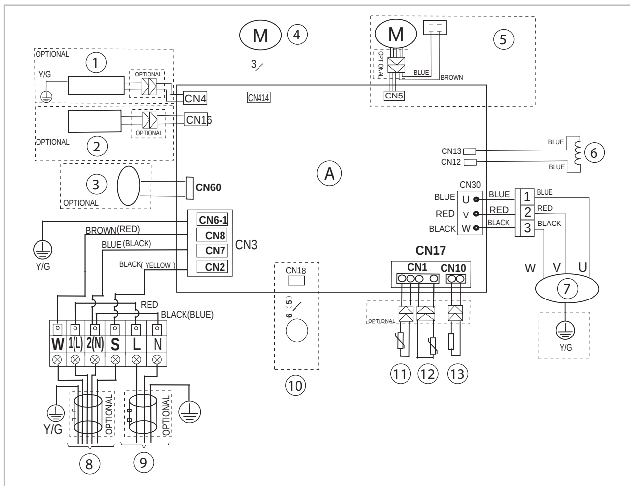
Abb. 39: Elektrisches Schaltschema RVT 265-355 ARCTIC AT
