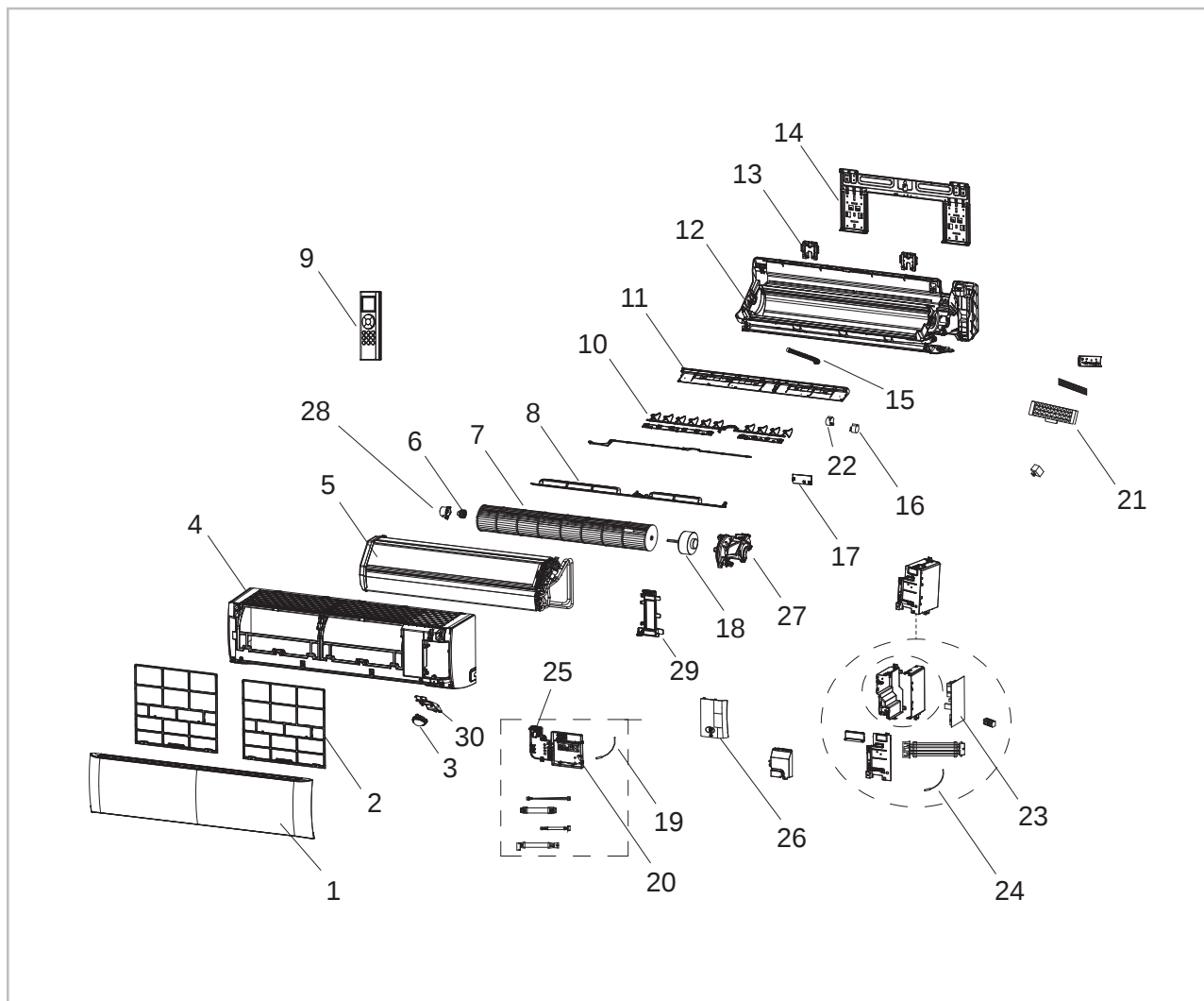
Abb. 45: Gerätedarstellung RVT 265-355 ARCTIC IT
