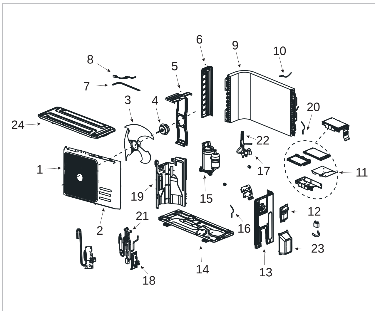
Abb. 46: Gerätedarstellung RVT 265-355 ARCTIC AT
