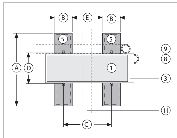
Abb. 33: Bemaßung des Streifenfundaments (Draufsicht)
