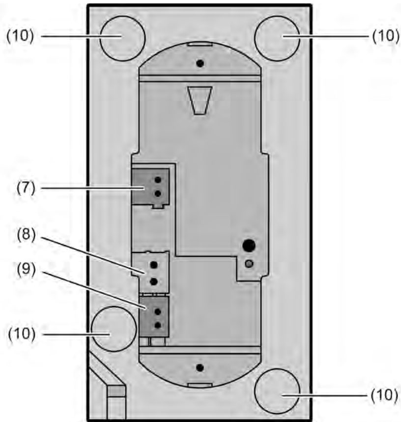
Bild 3: Geräteaufbau Rückseite
