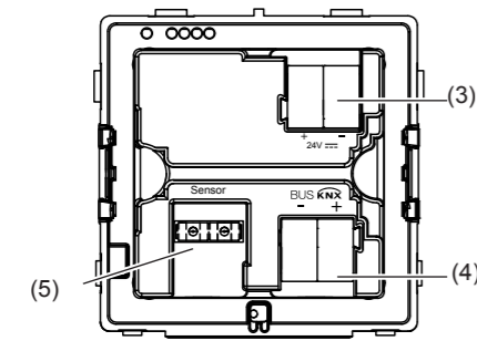
Bild 2: Rückansicht
