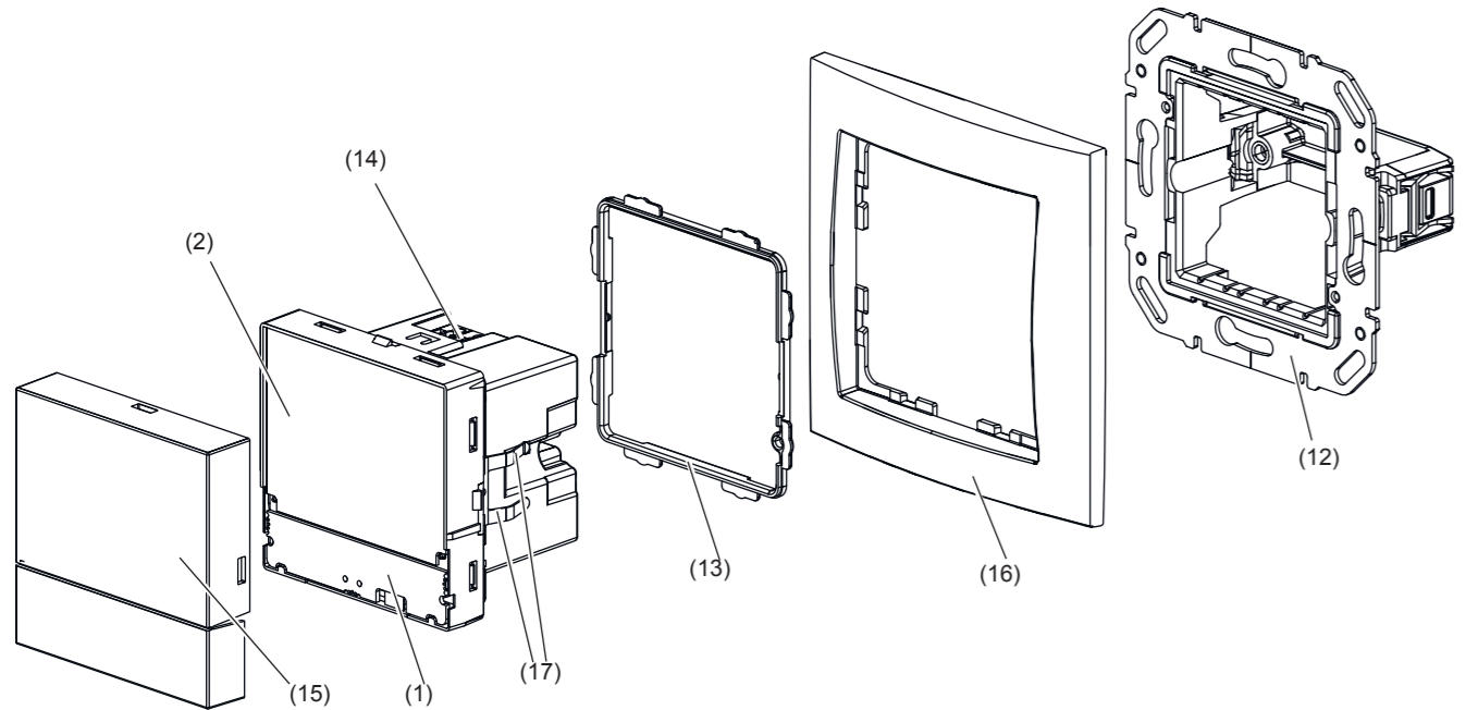
Bild 21: Gerät montieren
