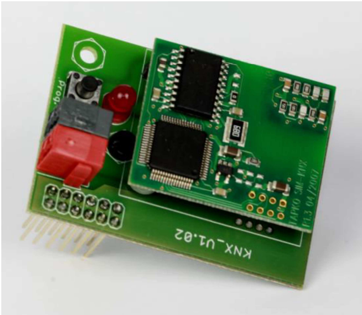
Abbildung 2: KNX-Modul
